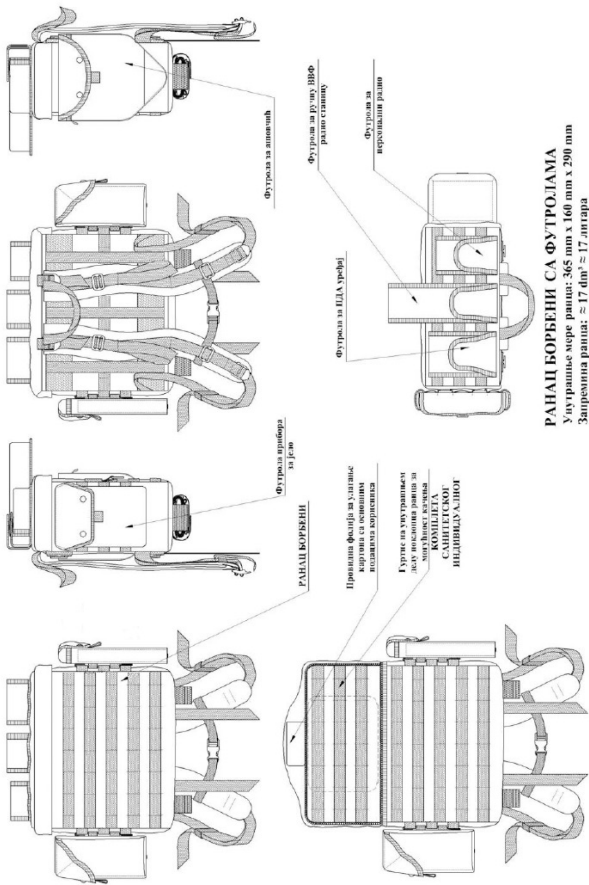
Слика 3. Изглед ранца борбеног са припадајућим футролама (није приказана футрола за санитарски комплект)
