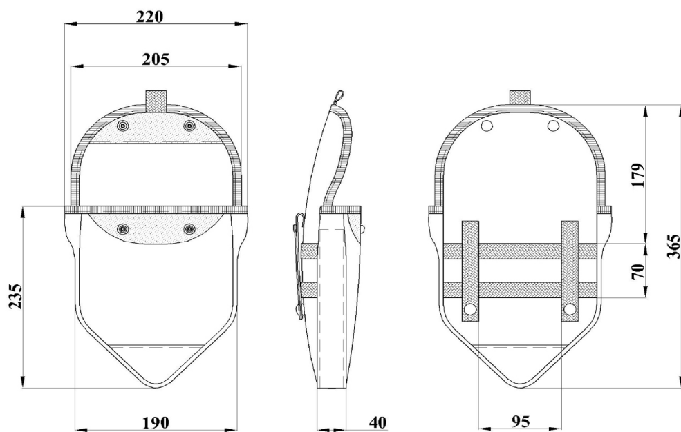
ФУТРОЛА ЗА АШОВЧИЋ
