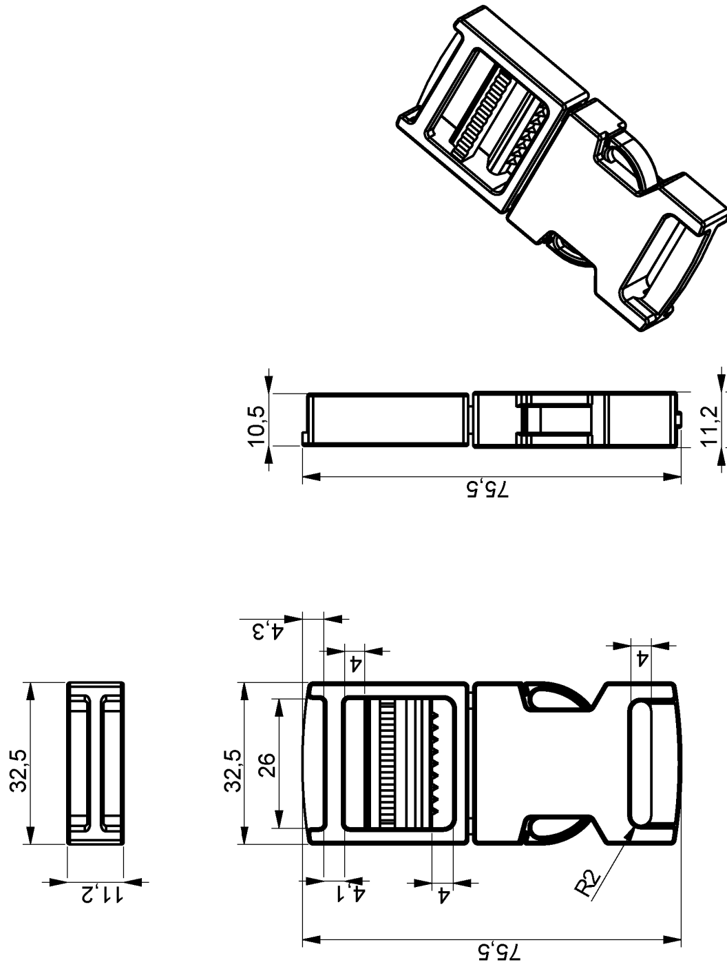
Слика 9. Изглед и димензије бравице за гуртну ширине 2,5м
